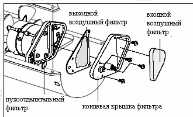
Рис. 10 Входной и выходной воздушные фильтры, фильтр пуха
