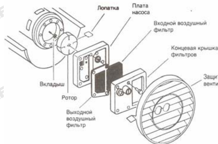
Рис.14 Расположение ротора
