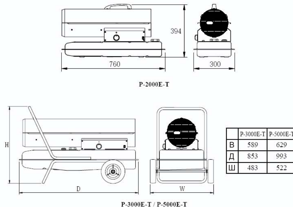
Рис.3. Нагреватель P-3000E-T, P-5000E-T
