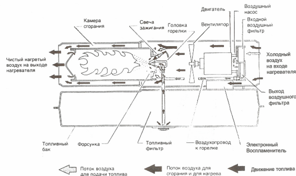
Рис. 5 Принцип работы
