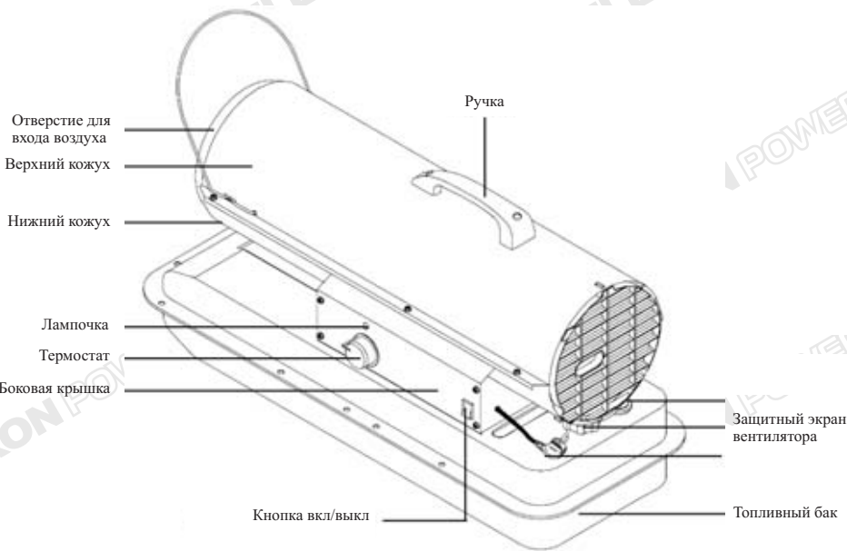
Рис. 1 Нагреватель P-2000E-T
