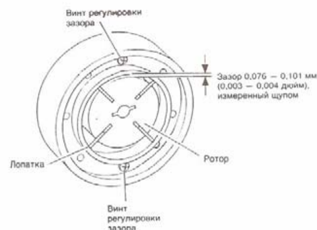
Рис.15 Расположение винтов регулировки зазора
